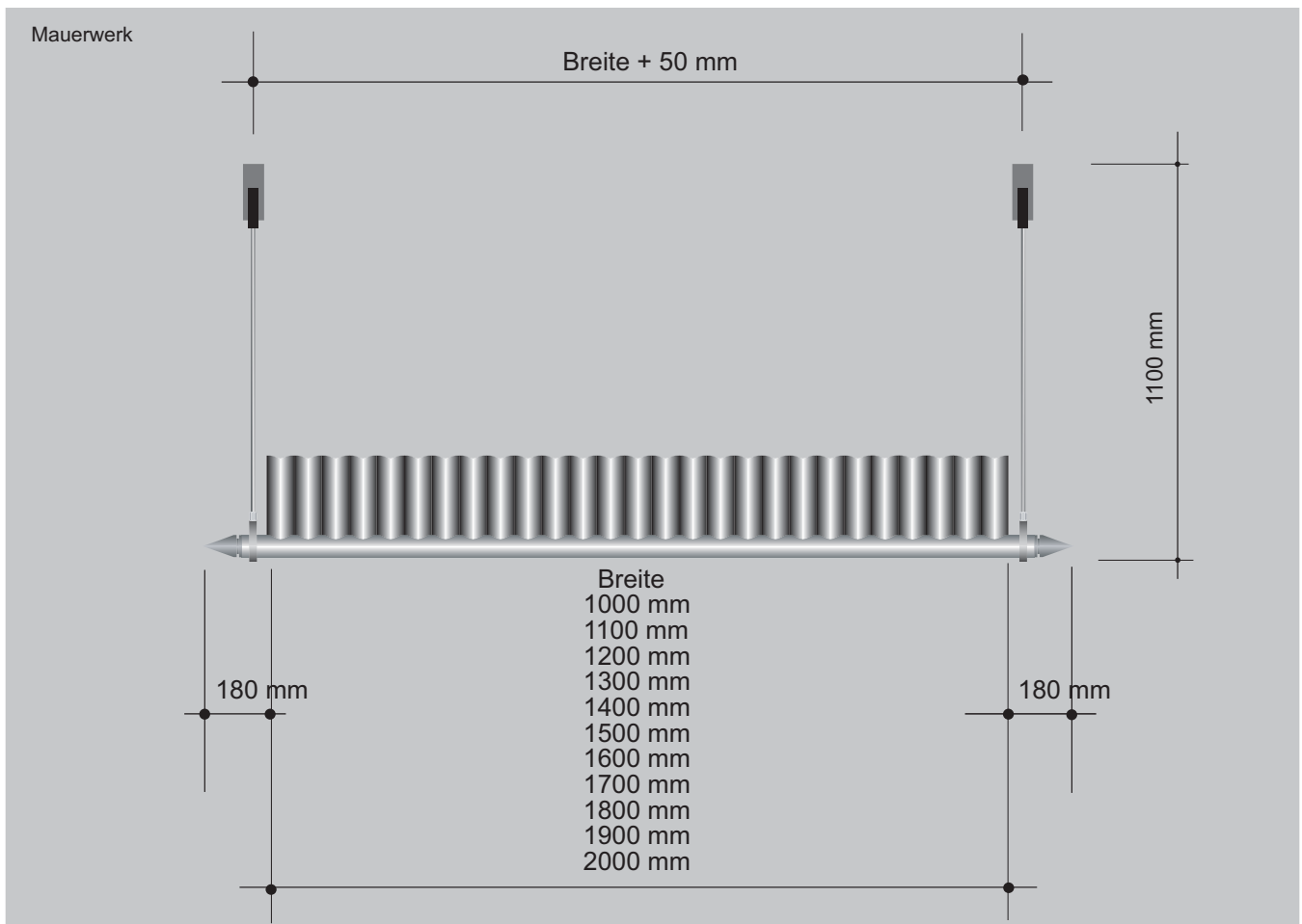
Vorderansicht
